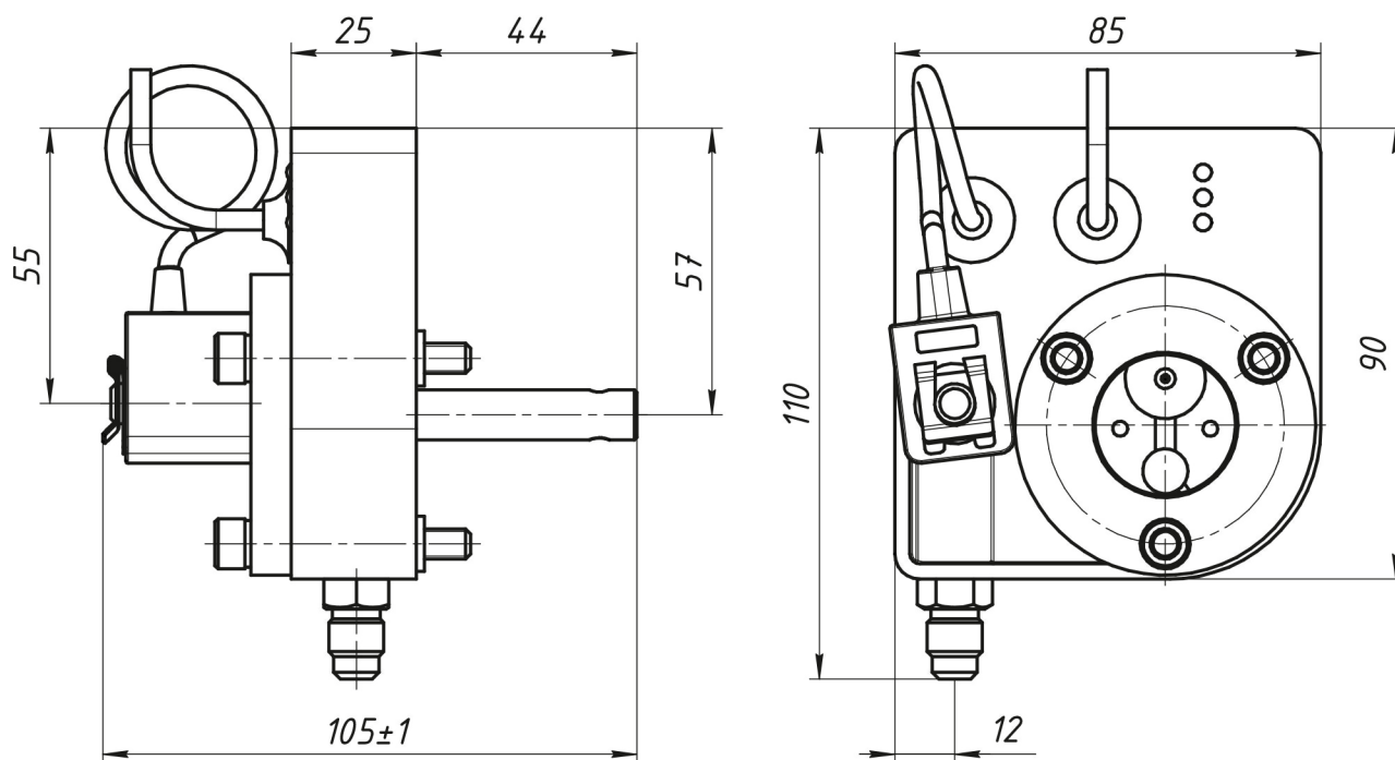
Fig.4. Dimensions
