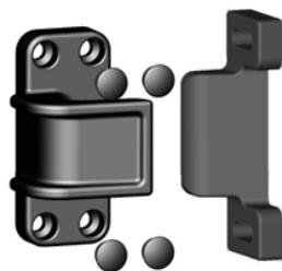
Guide fermeture Closing guide
