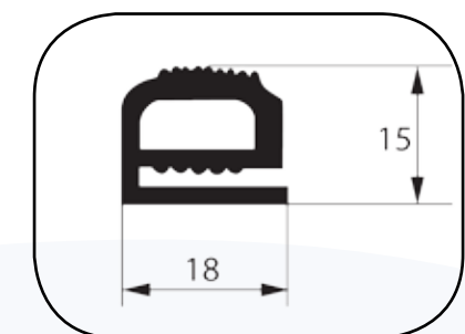
41 סיליקון -45°C / +50°C
