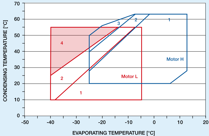
R22 APPLICATION LIMITS / LIMITI DI APPLICAZIONE R22
