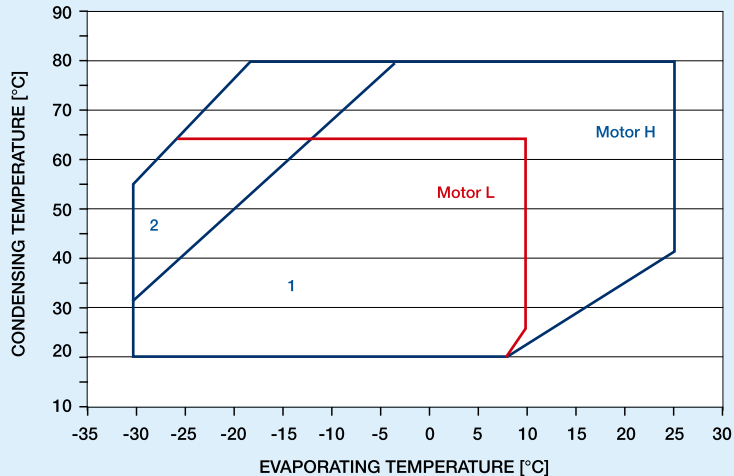
R134a APPLICATION LIMITS / LIMITI DI APPLICAZIONE R134a
