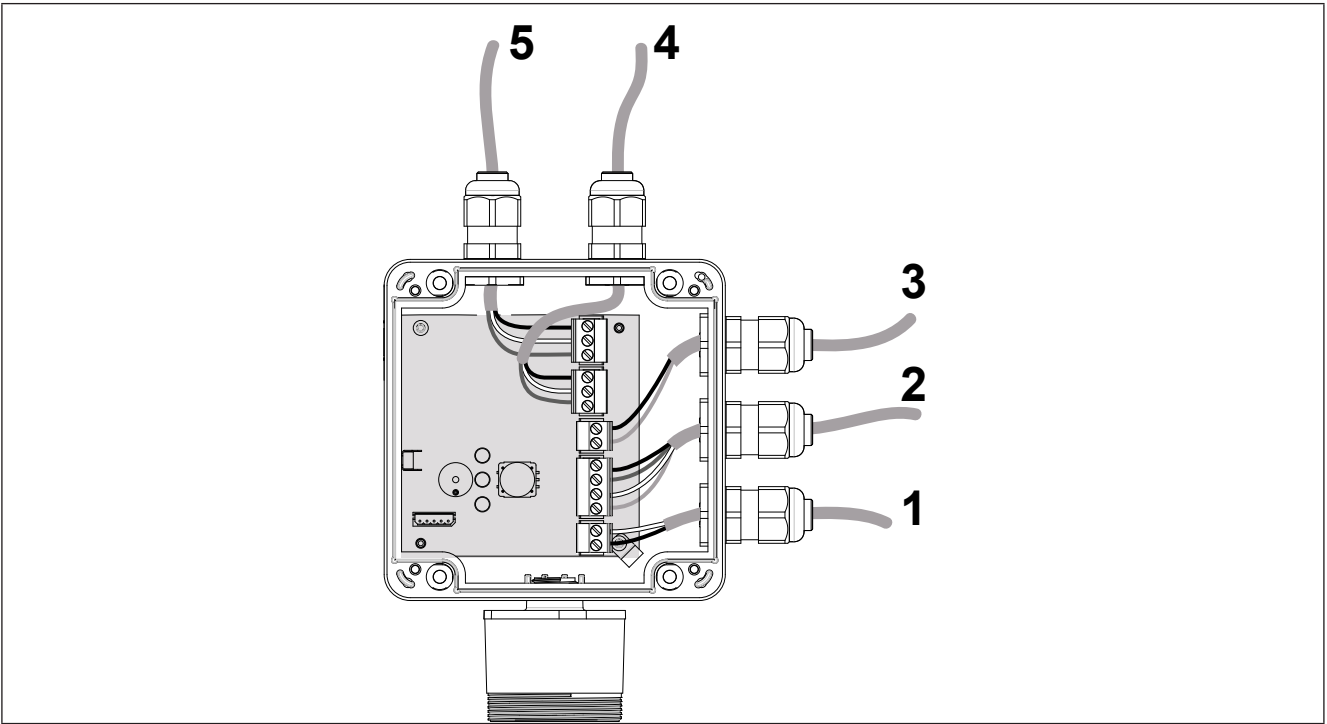
Fig. 16. Cable glands Wiring Best Praticce LKDNext
