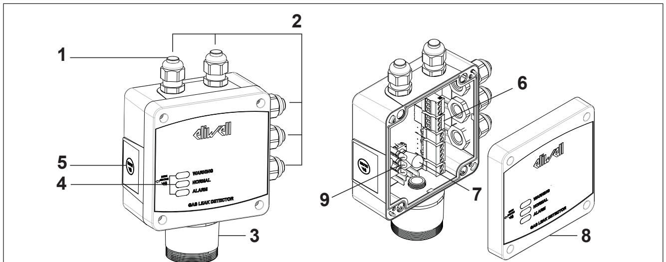
Fig. 2. LKDNext Components
